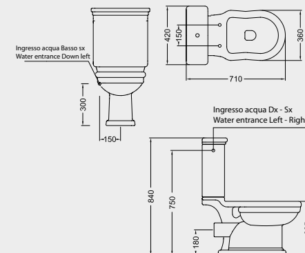
D13 VASO MONOBLOCCO SCARICO PARETE + D18 CASSETTA CERAMICA FUNZIONA CON 6 LITRI CLOSE-COUPLED WC "P" TRAP + CERAMIC MONOBLOCK CISTERN NOMINAL FLUSH 6 LITERS
