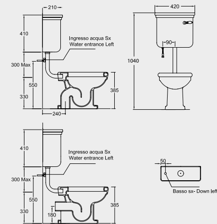
D23 CASSETTA CERAMICA A ZAINO LOW LEVEL CISTERN
