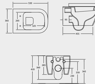
FAW10 VASO SOSPESO FUNZIONA CON 4,5 LITRI WALL HUNG WC NOMINAL FLUSH 4,5 LITERS
