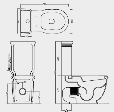
D23 CASSETTA CERAMICA A ZAINO LOW LEVEL CISTERN
