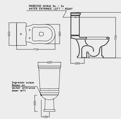
D12 VASO MONOBLOCCO SCARICO PAVIMENTO + D18 CASSETTA CERAMICA FUNZIONA CON 6 LITRI CLOSE-COUPLED WC "S" TRAP + CERAMIC MONOBLOCK CISTERN NOMINAL FLUSH 6 LITERS
