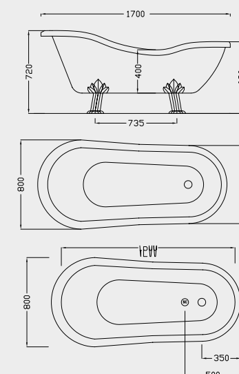
D60 - D61 - D62 - D63 VASCA BATHTUB
